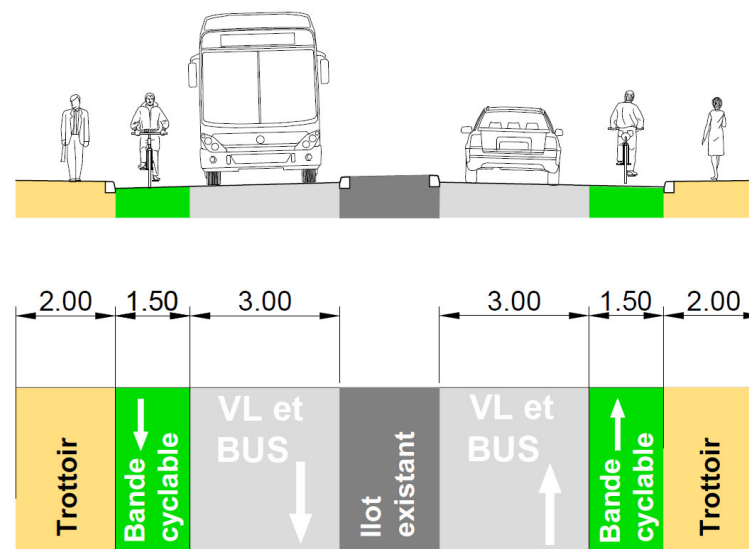
Emile Barneoud- coupes projet ZENIBUS – Bandes cyclables
